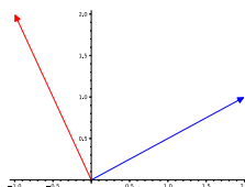
Figure 10.29. Les vecteurs \vec{u} et \vec{v}
