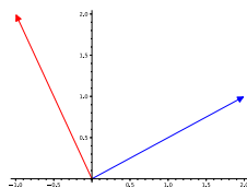
Figure 10.25. Les vecteurs \vec{u} et \vec{v}
